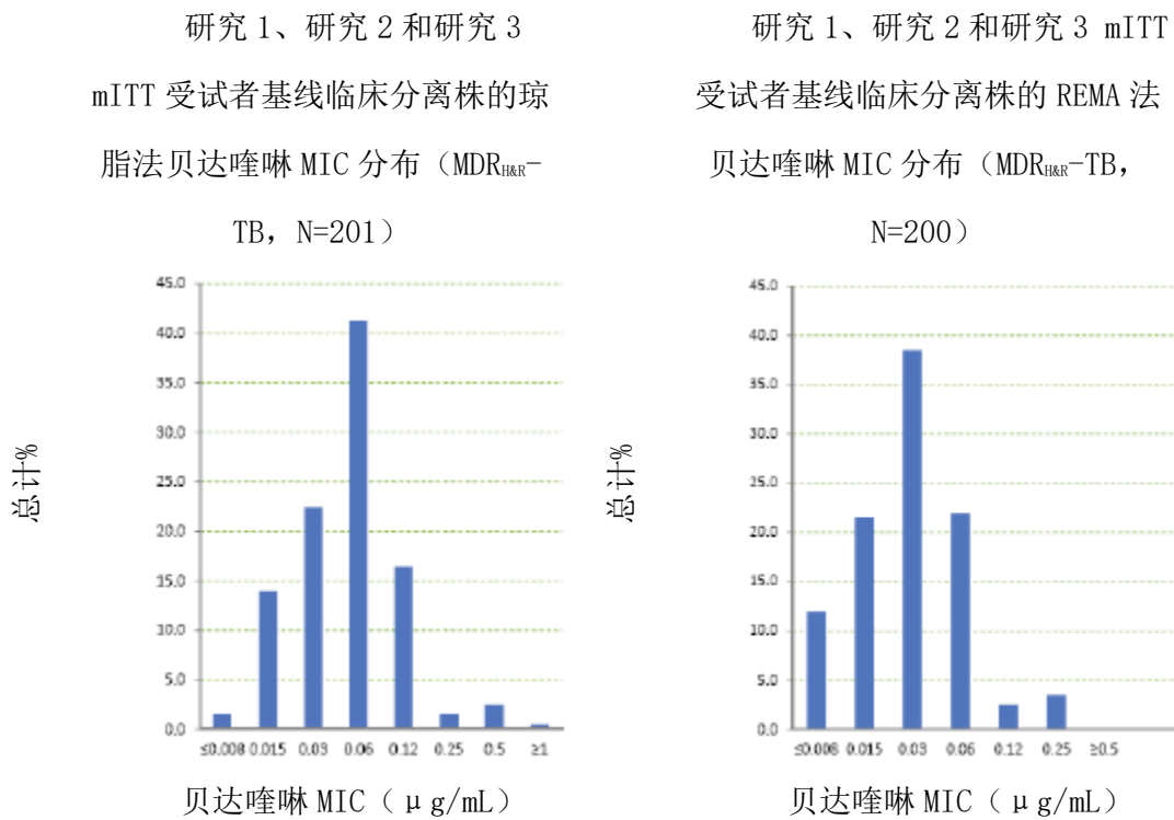
图 1：研究 1、2 和 3 mITT 成人受试者基线 MDR HR -TB 分离株的贝达喹啉 MIC 分布：琼脂法（左侧）和肉汤法（REMA）（右侧）
